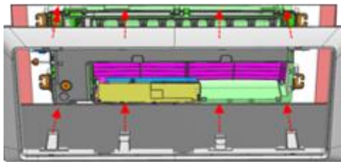
인테리어핏 패널 설치 (Screw 체결 없음/본체와 후크결합방식)
