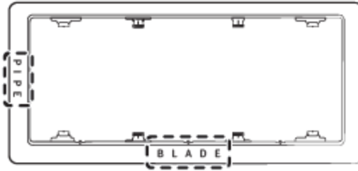
인테리어핏 패널 설치 방향 확인 (Blade부와 Pipe부 각인)
